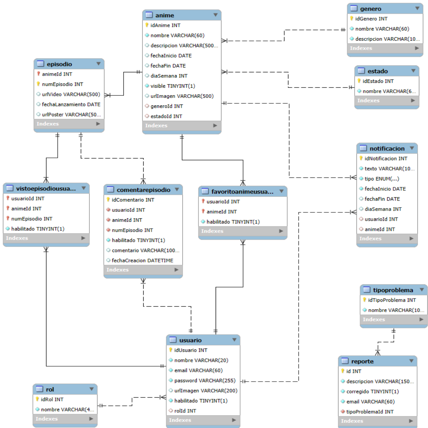
Ilustración 1 Diagrama Lógico
